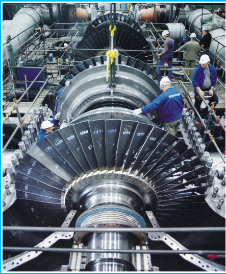
Imagem3- Engenharia mecânica
